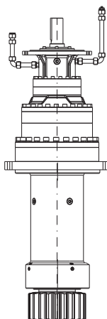
轴(电机)输入, 竖直安装
